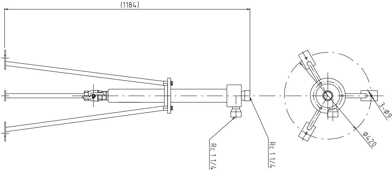
【アソカー取付図】
